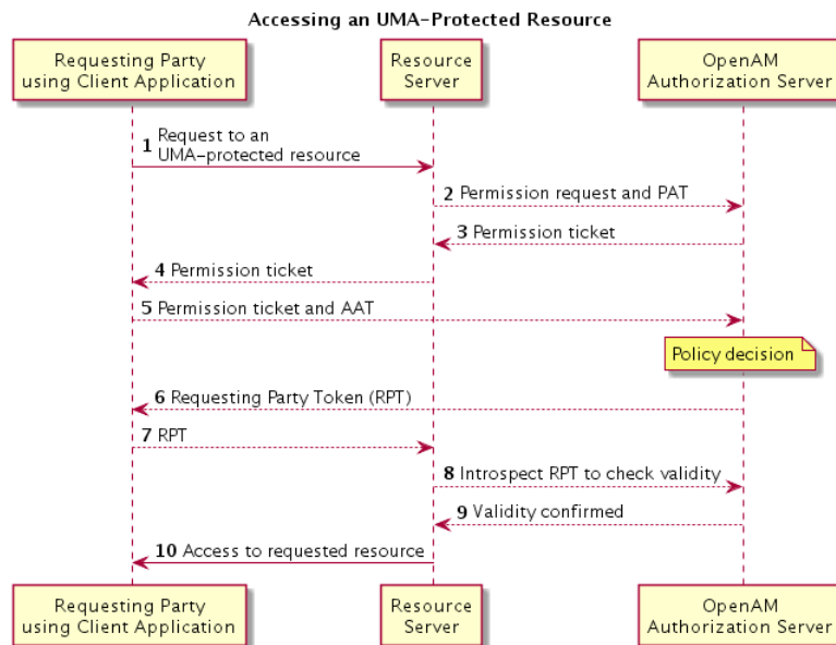
Figure 15.5. OpenAM in UMA RPT Token Flow
