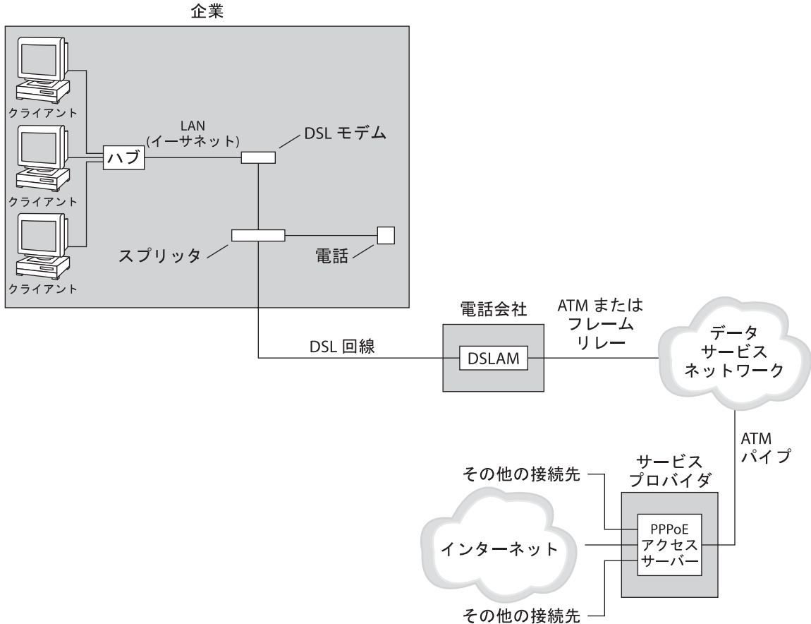
図 15-4 PPPoE トンネル内の関係者
