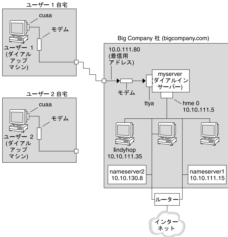
図 16-1 ダイアルアップリンクの例
