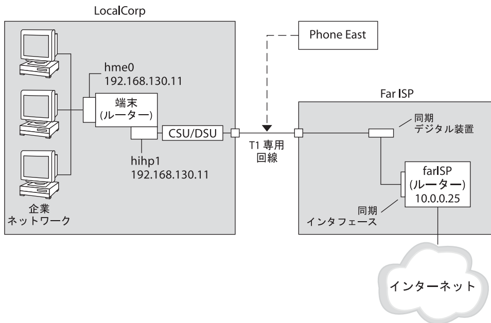
図 16-2 専用回線の構成例
