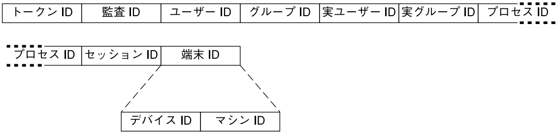
図 31-5 process トークンの形式
