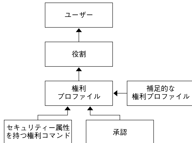
図 8-1 Solaris RBAC 要素の動作
