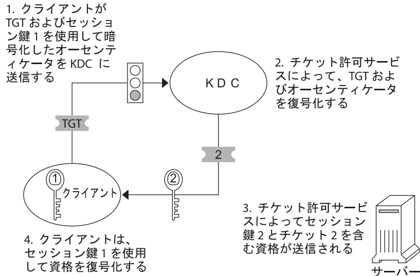
図 27-3 サーバーに対する資格の取得
