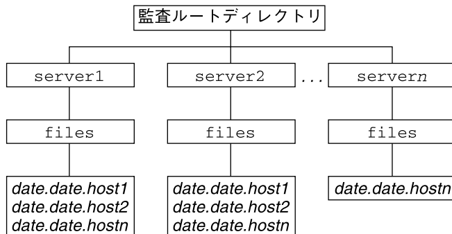
図 31-2 サーバーごとに格納された監査トレール
