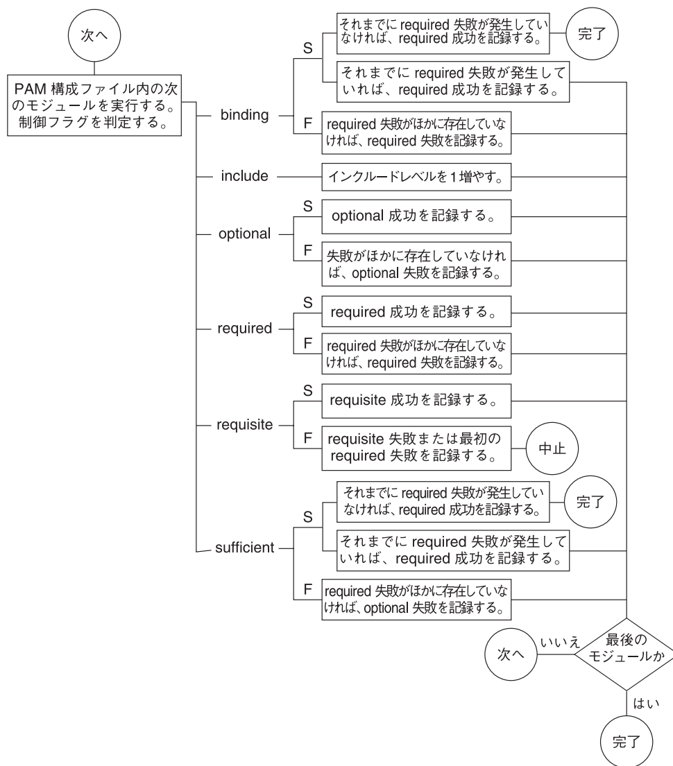
図 17-2 PAM スタック: 制御フラグの効果
