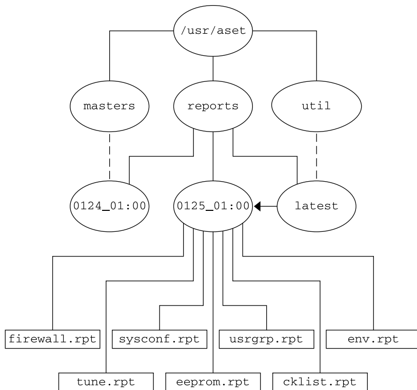
図 7-1 ASET reports ディレクトリの構造
