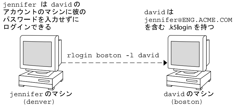
図 26-1 アカウントへのアクセスを認可する .k5login ファイルの使用
