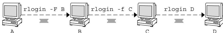
図 26-3 転送可能チケットの使用
