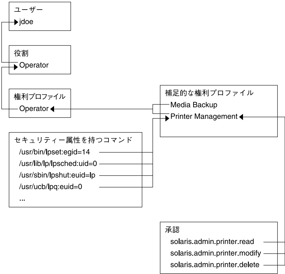
図 8-2 Solaris RBAC 要素の関係の例
