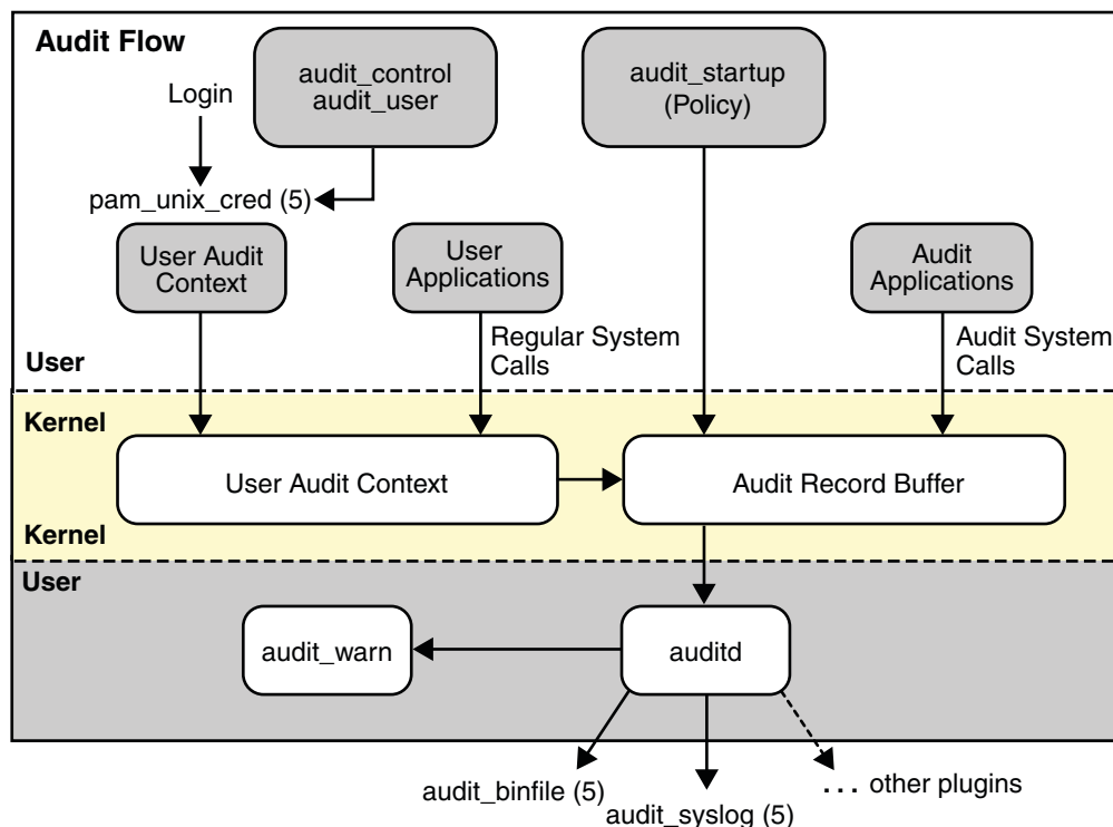
図 28-1 監査のフロー
