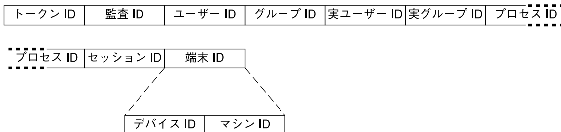
図 31-6 subject トークンの形式
