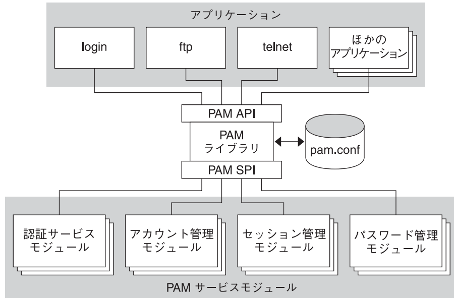
図 17-1 PAM のアーキテクチャ
