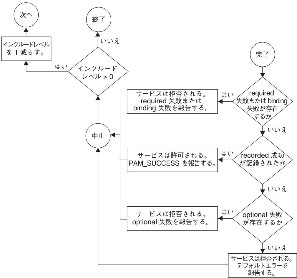
図 17-3 PAM スタック:統合された値の決定方法
