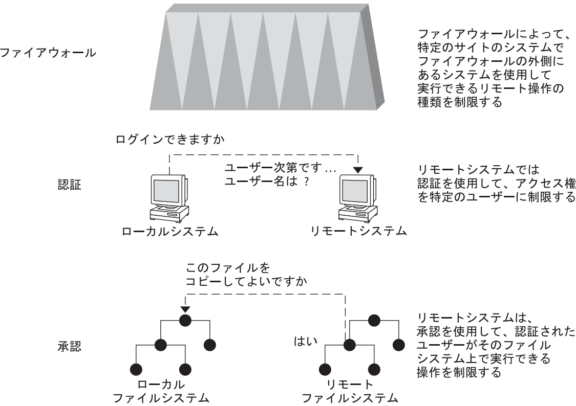
図 2-1 遠隔操作のセキュリティ制限
