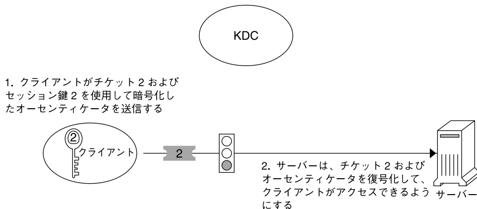
図 27-4 特定のサービスへのアクセス権の取得
