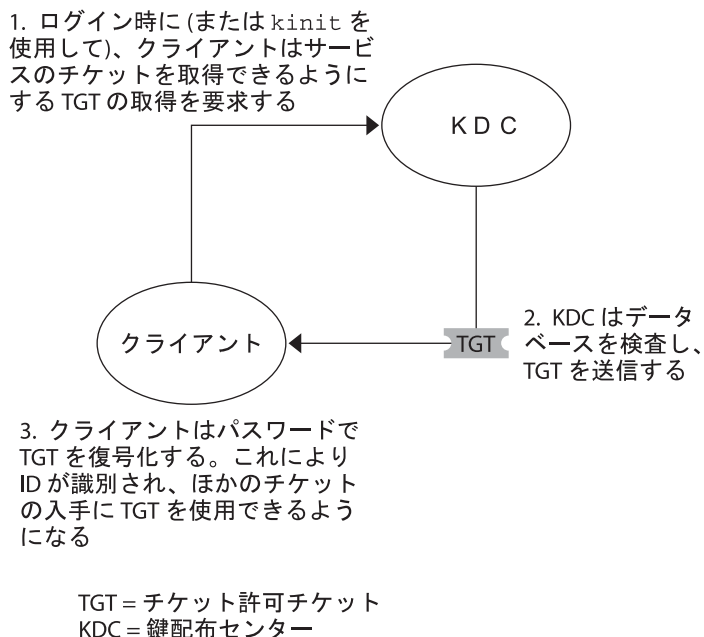
図 21-1 Kerberos セッションの初期認証
