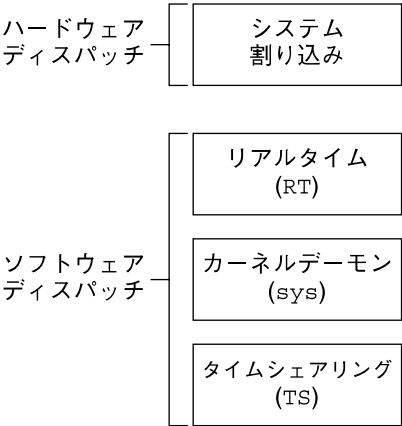
図 12-4 スケジューリングクラスのディスパッチ優先順位
