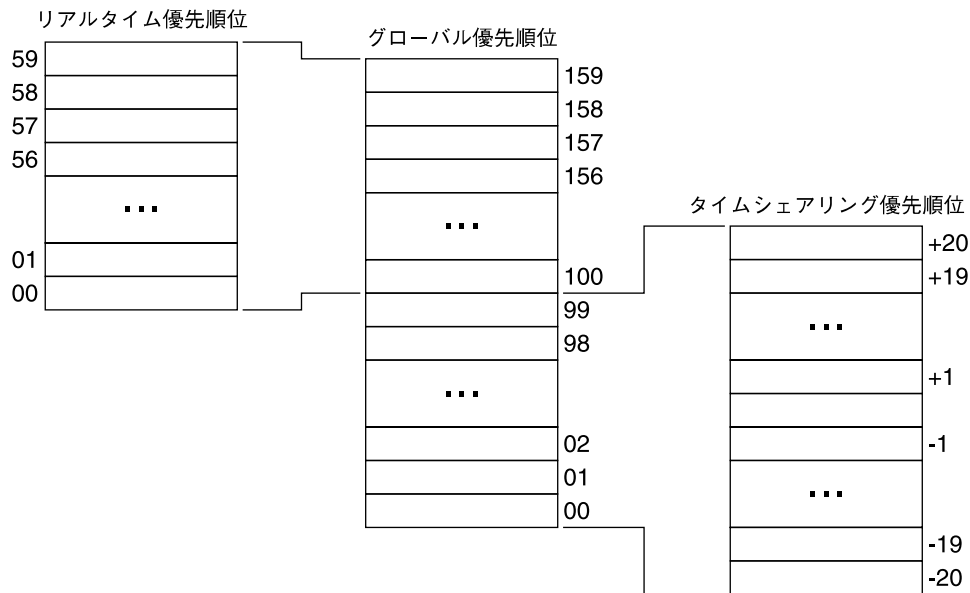
図12-5 カーネルディスパッチ待ち行列
